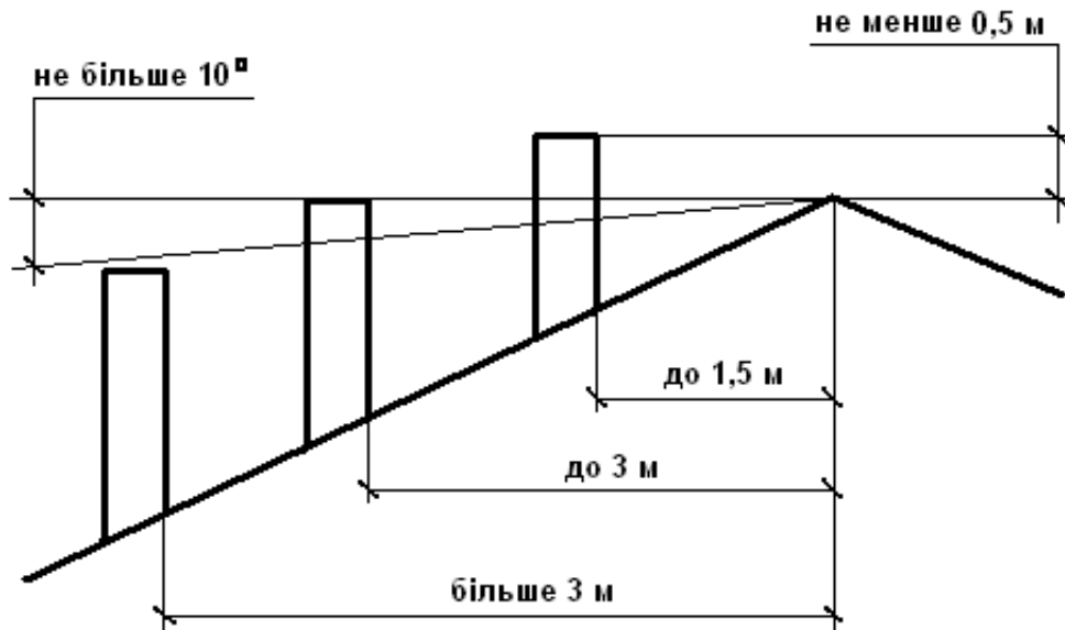
Рисунок 5. Розміщення димоходу
