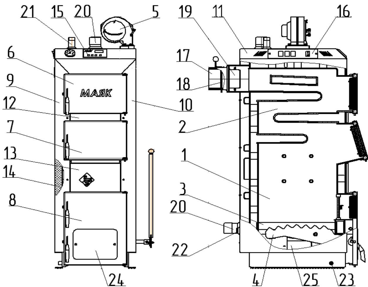
Рисунок 1. Котел опалювальний КТР-16 ECO MANUAL
