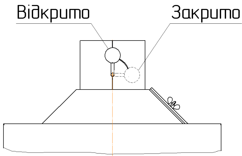
Рисунок 5. Регулювання положення шибера.
