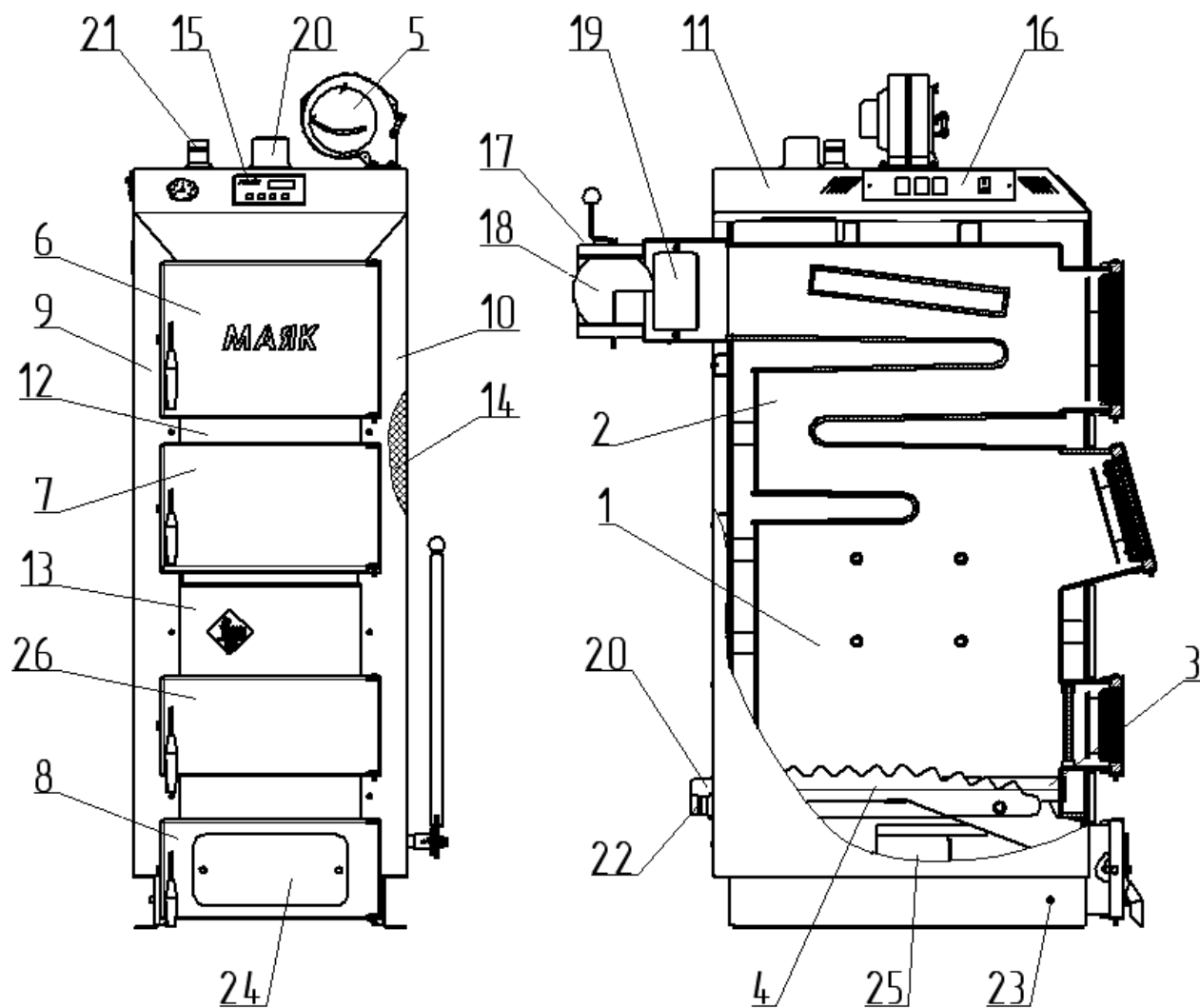
Рисунок 2. Котел опалювальний КТР-25 ECO MANUAL
