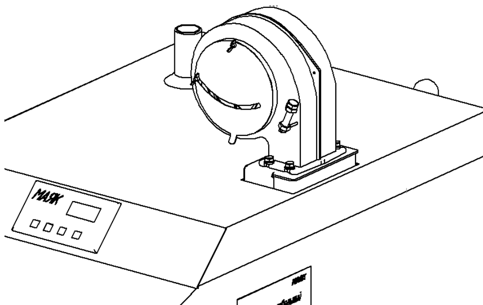
Рисунок 6. Монтаж вентилятора
