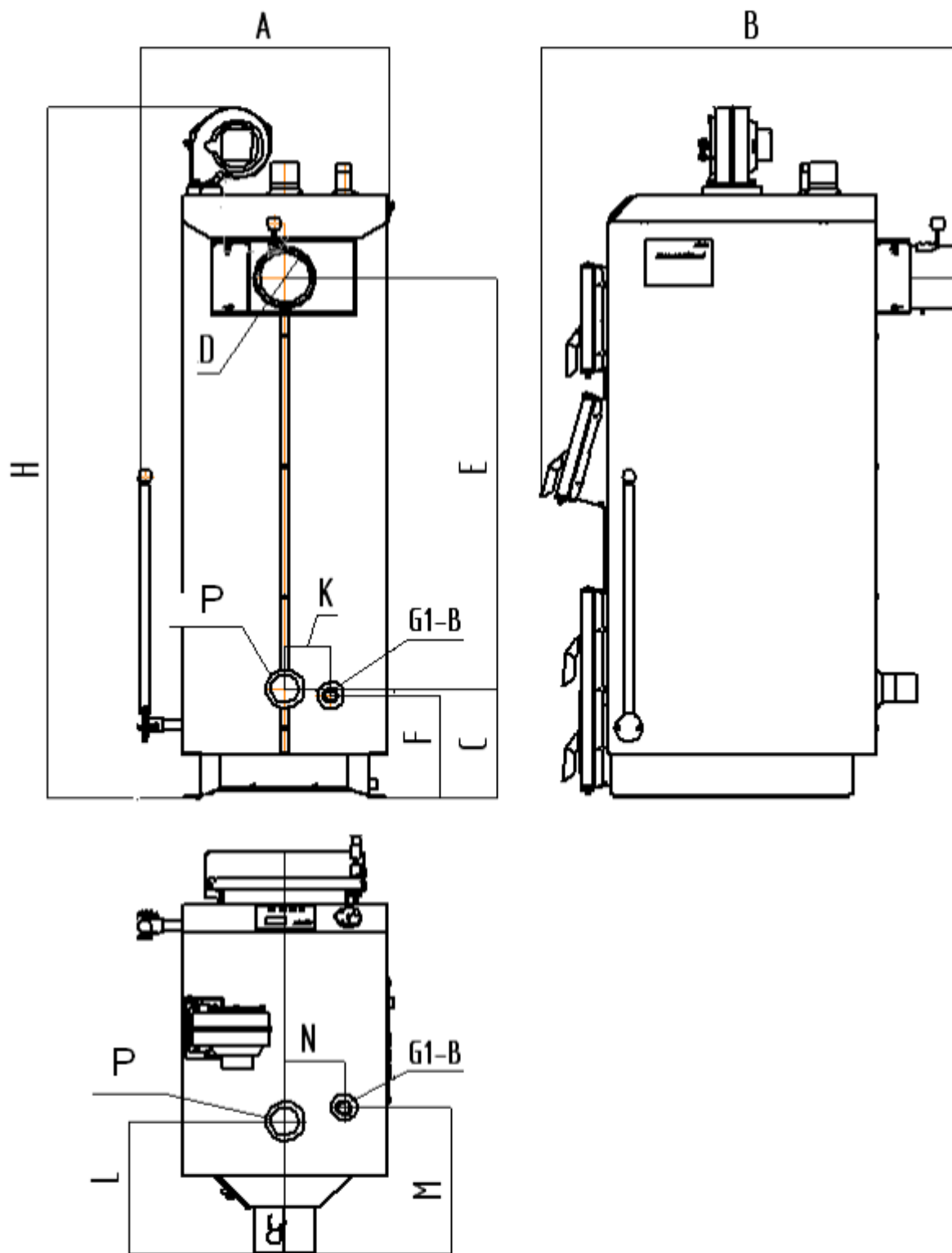
Рисунок 3. Приєднувальні розміри
