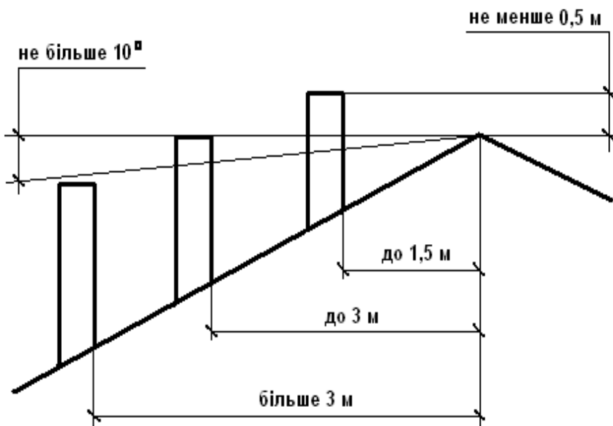
Рисунок 6. Розміщення димоходу
